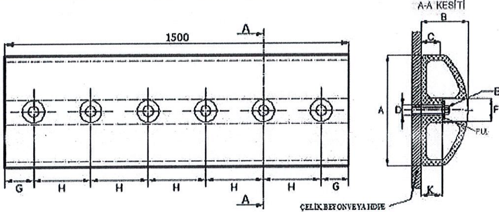
B TİPİ USTURMAÇA ÖLÇÜLERİ
